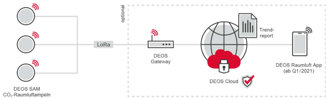
Topologie DEOS Raumlufttampel SAM
